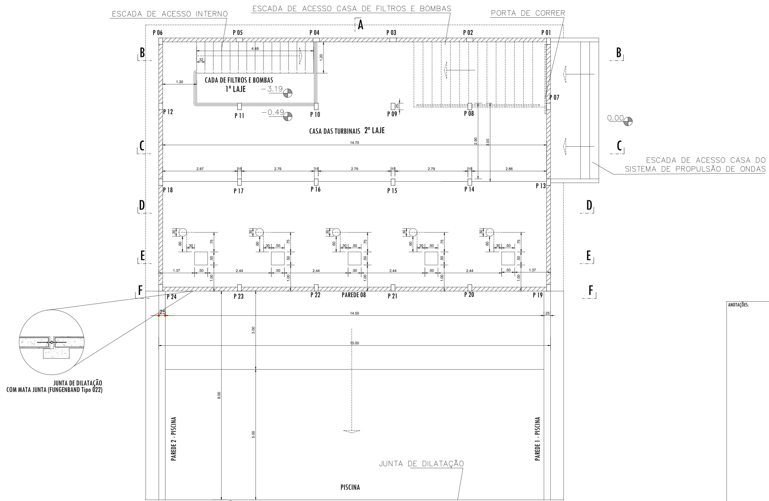
PLANTA "5" PISCINA COM ONDAS
