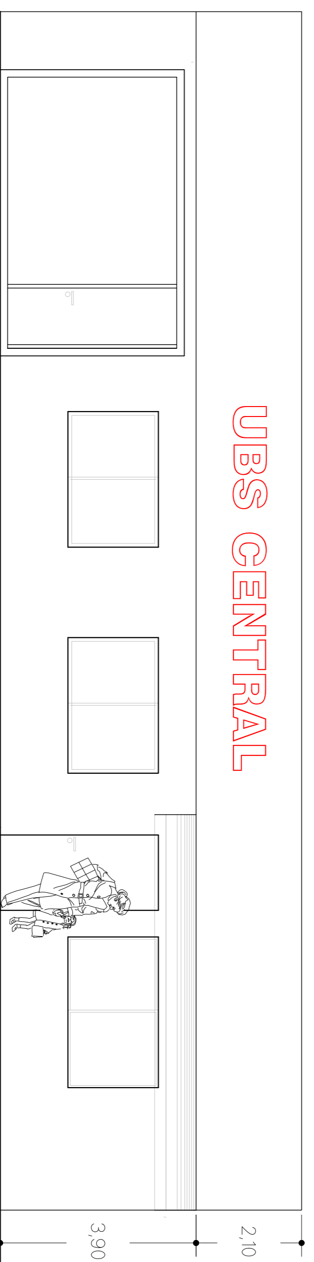
FACHADA FRONTAL
