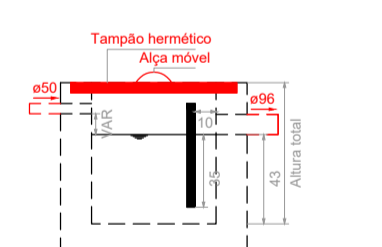
Caixa de gordura - TÉRREO Corte 1 - ESC. 1:25
